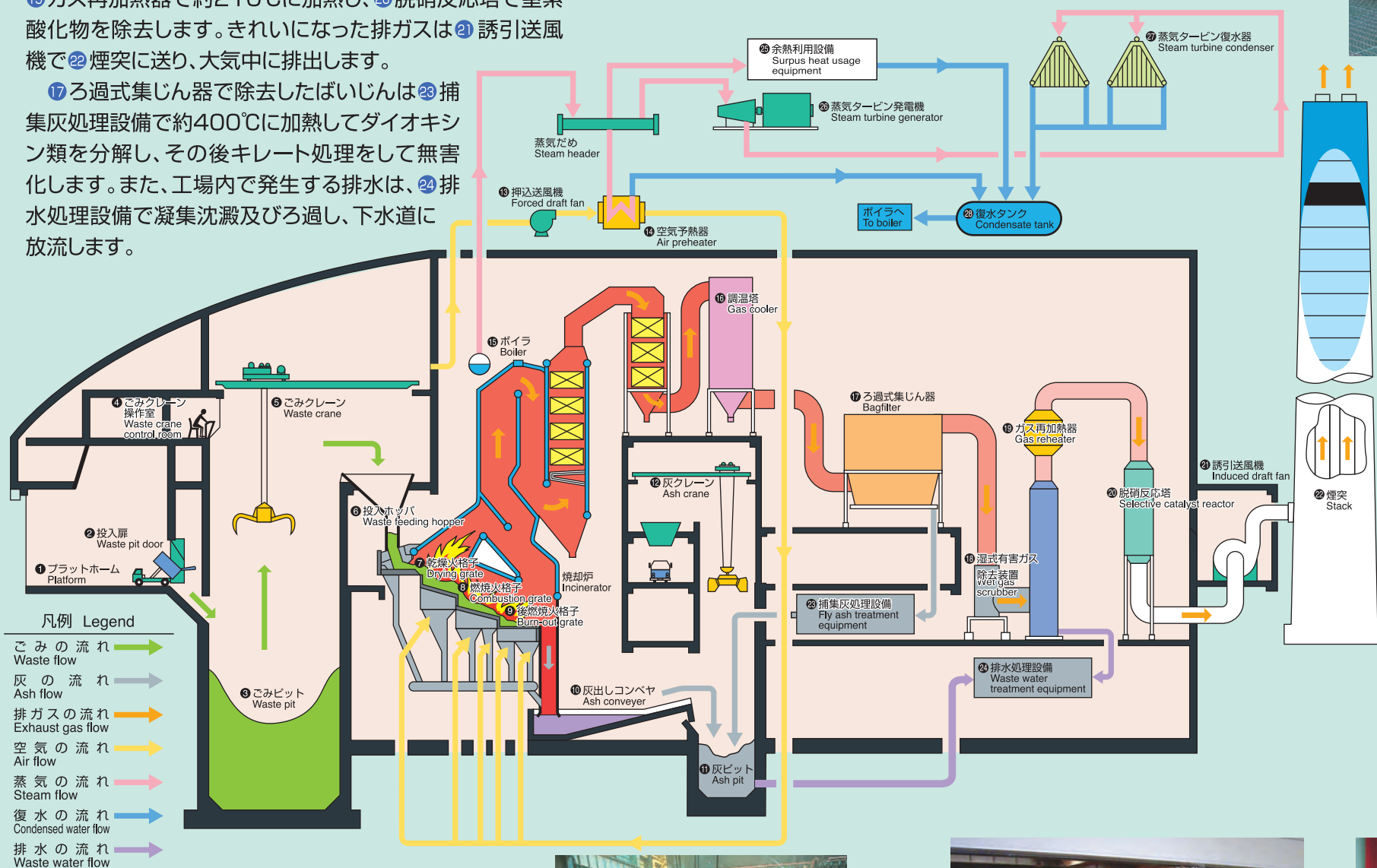
ボイラ 焼却熱を利用し、蒸気を発生させます。 Boiler: Uses garbage heat to generate steam.
