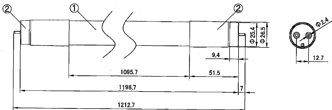
【種別】直管LEDランプ 32形
