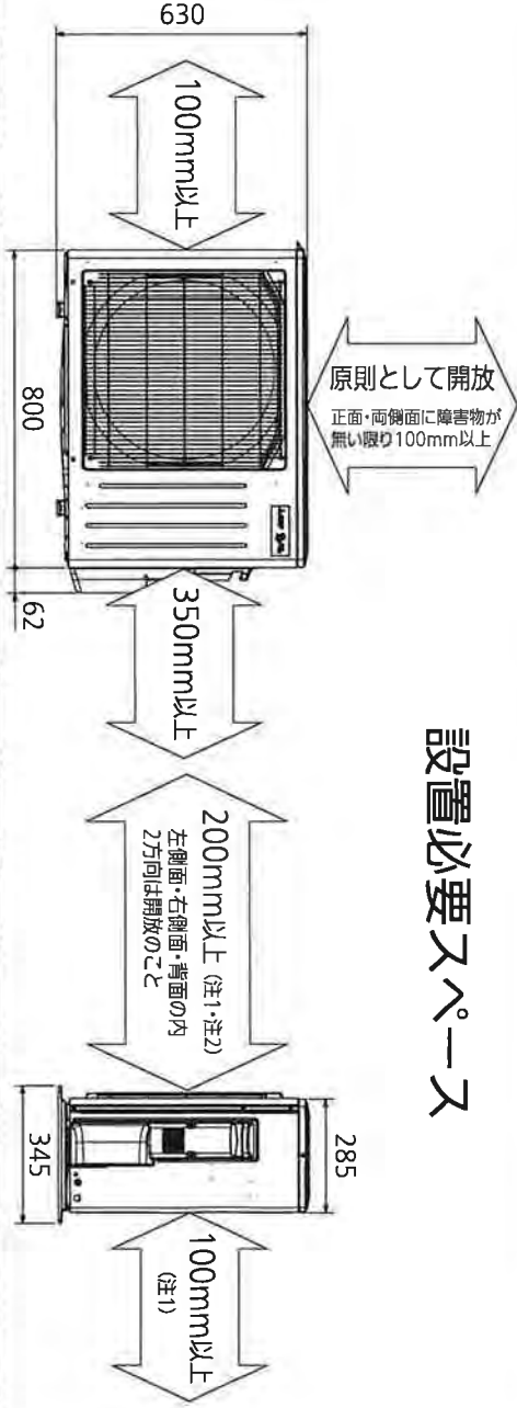
(平面図)
