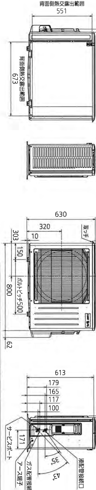
(正面図)
